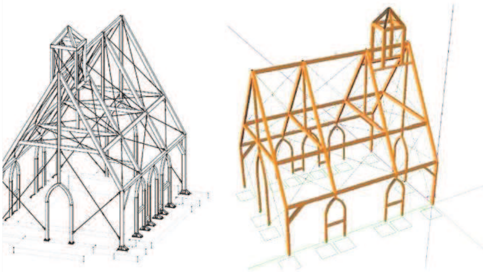
Jedna z wizualizacji przedstawiająca współczesną rekonstrukcję bryły kościoła w Warzymicach
