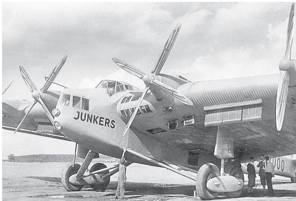
Pasażerski Junkers Grossflugzeug G 38 (D-2000). Zdjęcie datowane na 1930 rok. Widoczne kabiny pasażerskie w skrzydłach
